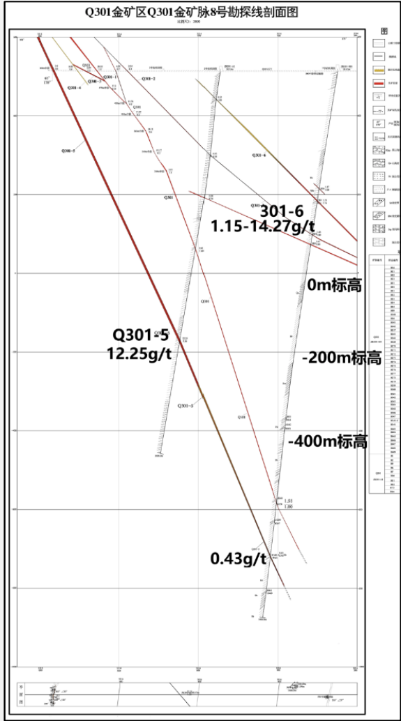
潼关301矿区8勘探线剖面图
