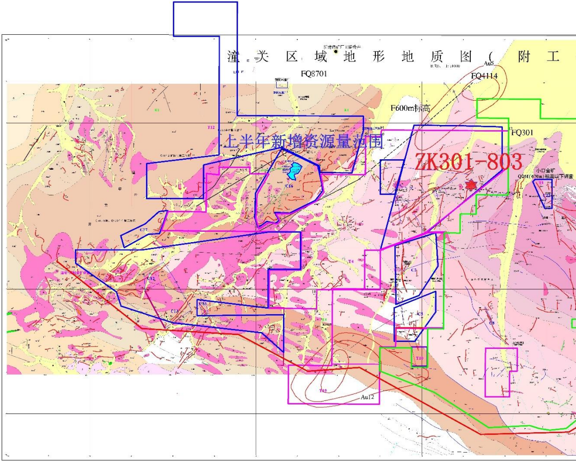
潼关地区地质平面图
