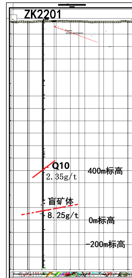
北东金矿22勘探线剖面图
